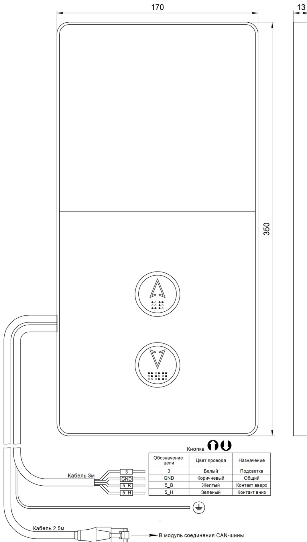
Рис.1 Внешний вид, габаритные и установочные размеры Вызывного поста МАЛАХИТ (жгут RJ45) НШЕК.468381.018
